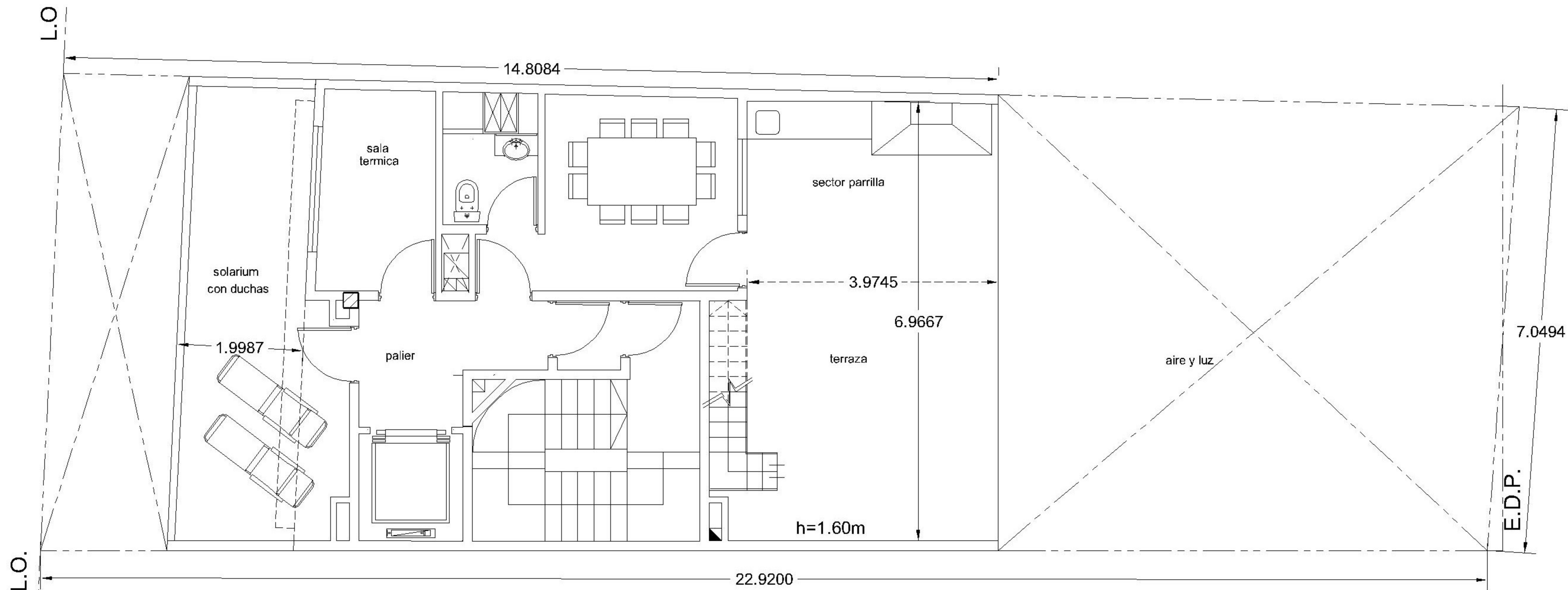
PLANTA 12 piso
